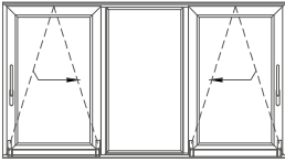
Scorrevole parallelo con ribalta, 3 componenti 1 SX / 1 DX
