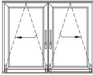
Scorrevole parallelo con ribalta 1 SX / 1 DX
