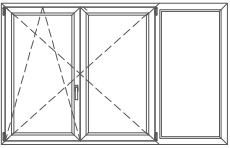
Finestre con fiancoluce fisso
