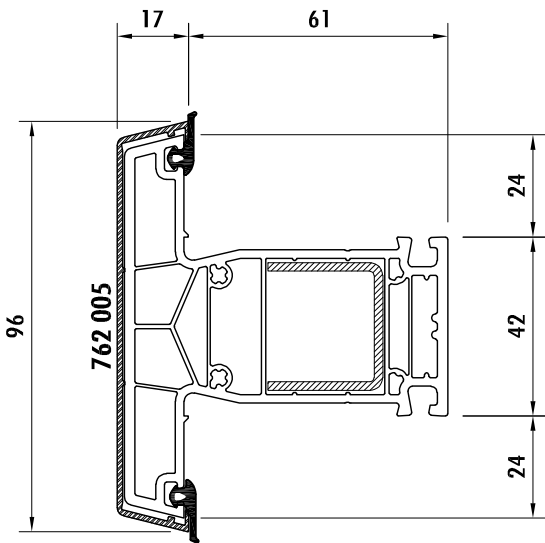
PIANTONE/TRAVERSO PER ANTA 762 005 per abbinamento vetro
