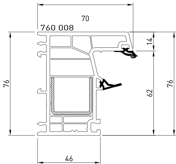
Telaio piano 760 008
