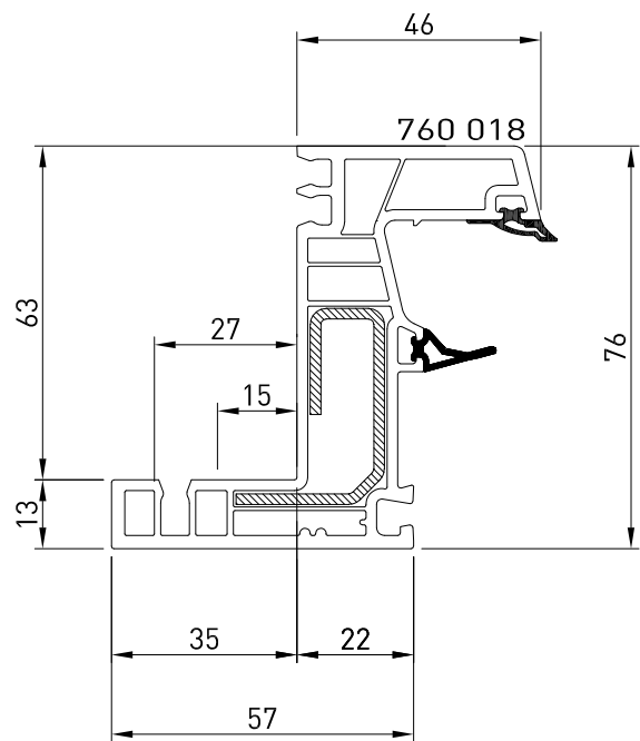
Telaio Z con aletta da mm 35 760 018
