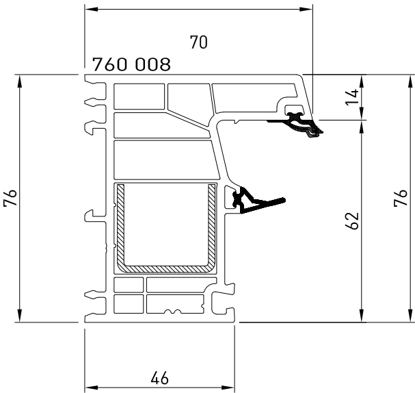
Telaio piano 760 008
