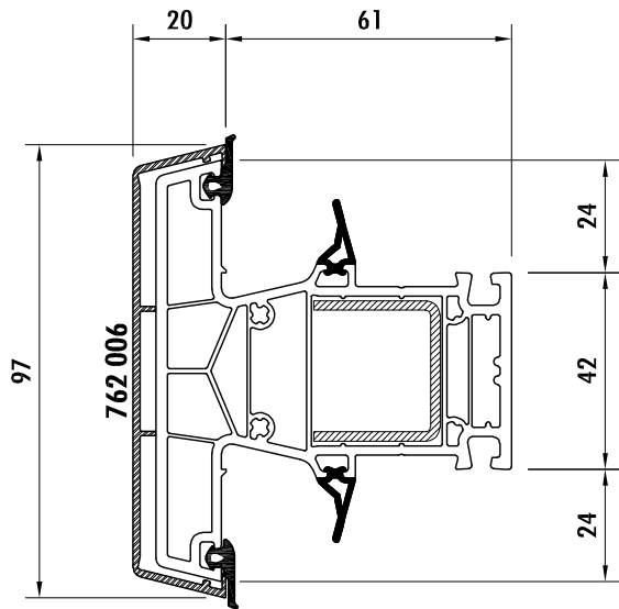
PIANTONE/TRAVERSO PER TELAIO 762 006 per abbinamento anta
