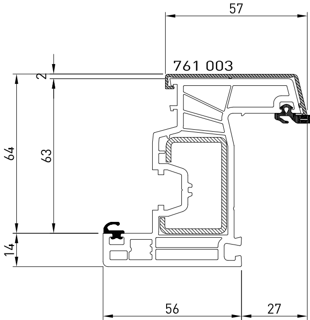
Anta 761 003
