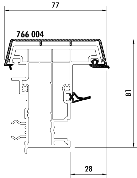
SCAMBIO BATTUTA 766 004
