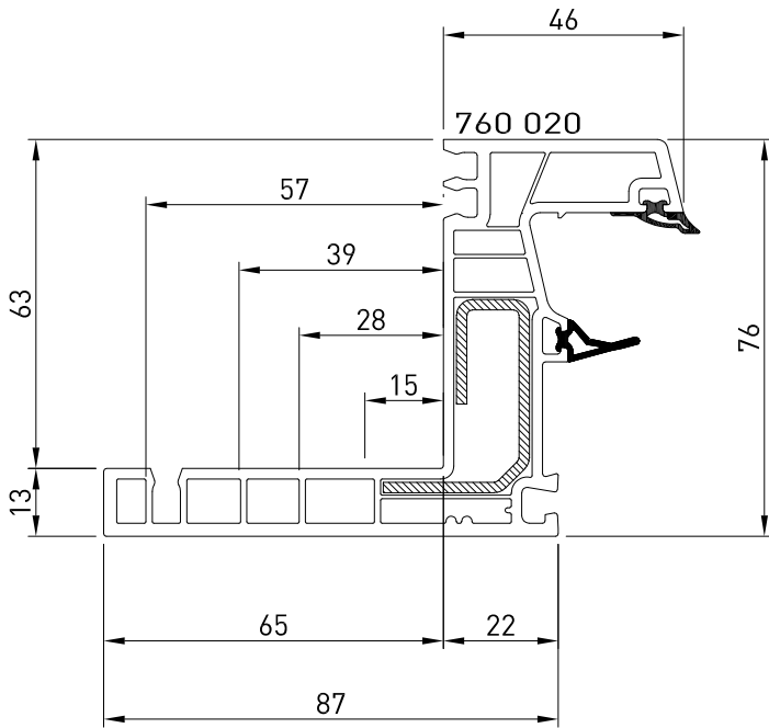
Telaio Z con aletta da mm 65 760 020
