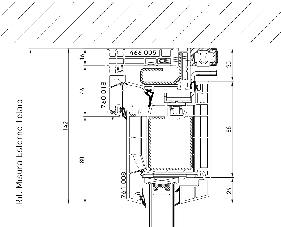
TAV. 3 TELAIO a Z con aletta da mm 35 760 018
