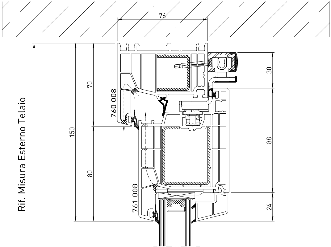
Nodo Superiore
