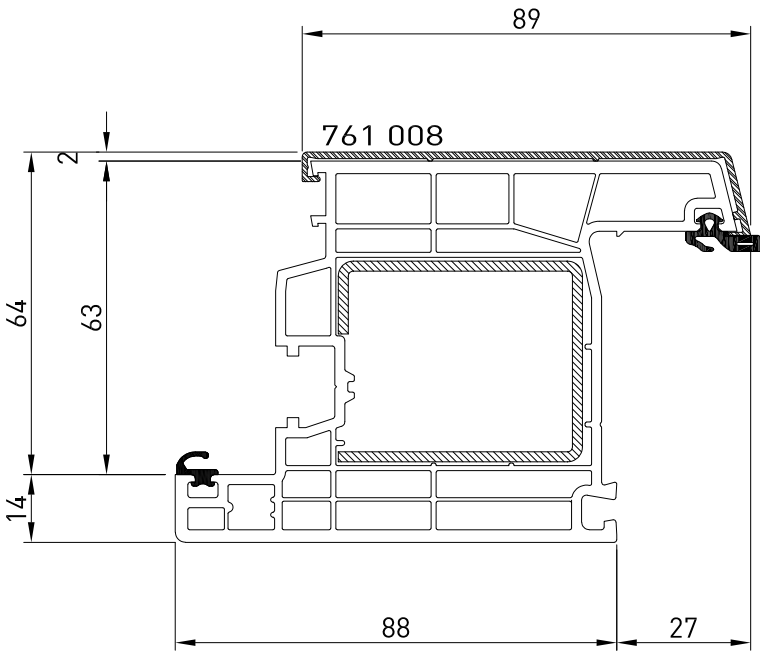
Anta Maggioreta 761 008
